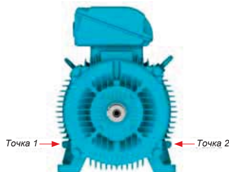
Рисунок 8 - Расположение клемм заземления в корпусе
