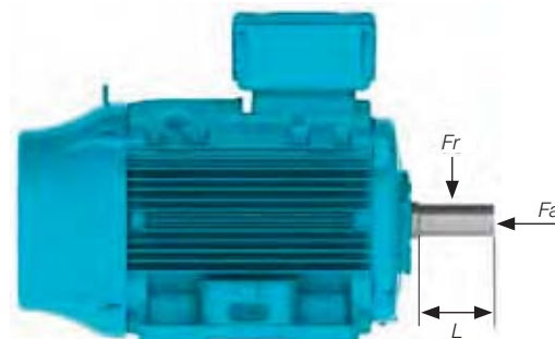
Рисунок 25 – Радиальная и осевая нагрузки на вал двигателя
