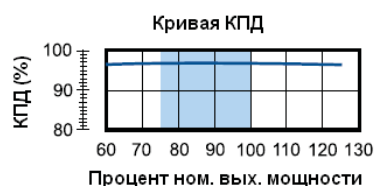
Рисунок 2 – Стандартная кривая КПД двигателей линии W22
